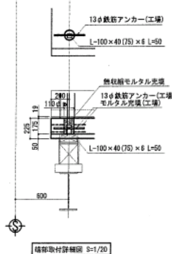
端部取付詳細図 S=1/20
