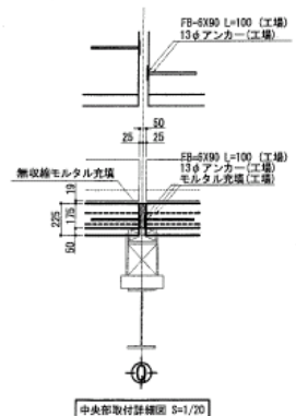
中央取付詳細図 S=1/20
